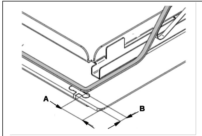
Afb. 8 Glas met lijst
