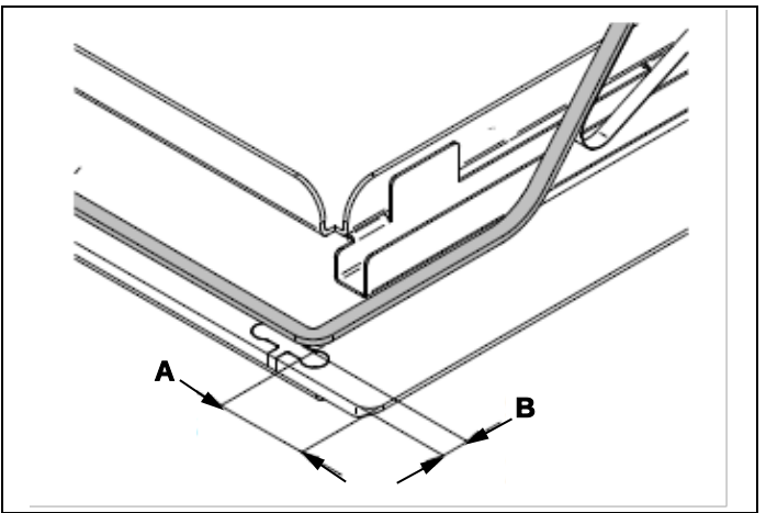
Fig. 8 Vetro con cornice
