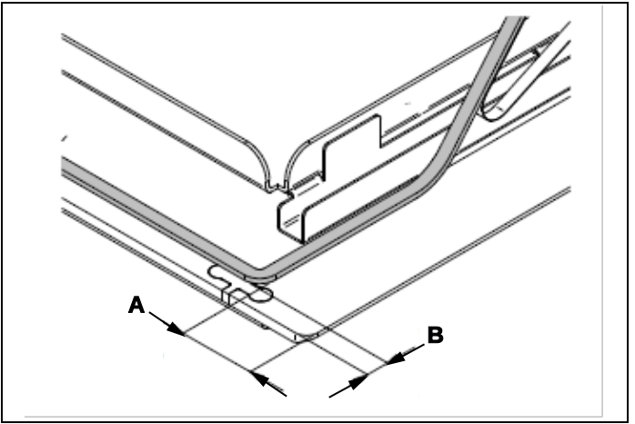
Fig. 8 Vitre avec cadre
